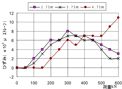
図 - 15 荷重 - ひずみ曲線 (図 - 14 の摩擦型アンカー体) (アンカー体より 25cm 離れた地盤内で測定)
