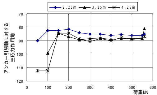
図 - 20 クサビ主応力方向(泥岩 = 1.1N/mm 2 ) (定着長 2m, 荷重作用点はクサビ中央)
