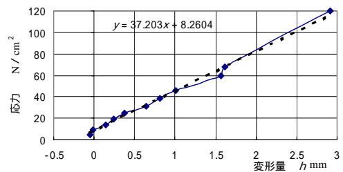
図 - 21 応力 - 変形量曲線(泥岩 = 1.1N/mm 2 )
