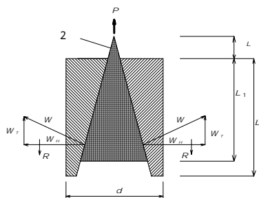
W_T クサビ接線力、 W ：クサビ力、 R ：摩擦抵抗 L ：クサビ長、 L_1 ：有効支圧区間長、 L_2 ：クサビ引抜け長
