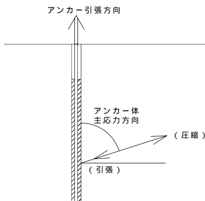
図 - 5 アンカー体主応力方向説明図
