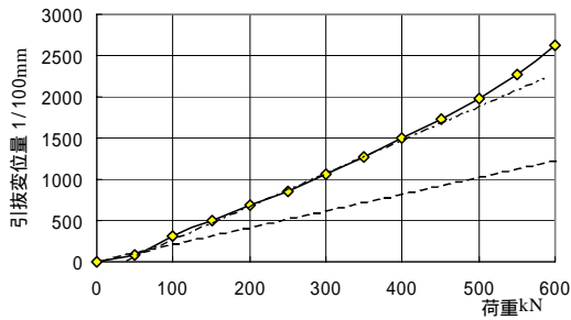
図 - 14 荷重 - 変位曲線 (マッツ型: 定着長 4.5m) (破線は理論伸び量)
