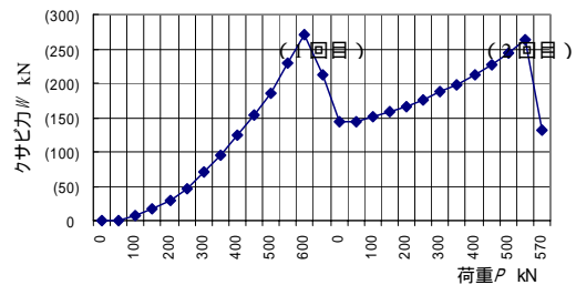
図 - 22 アンカー体の耐久性(泥岩 = 1.1N/mm 2 ) (クサビ力はアンカー体より 1m 地点のもの)
