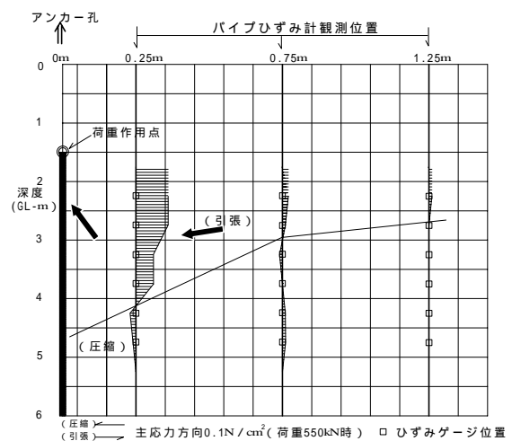
図-3 マサツ型アンカー体(引張)周辺地盤の応力図 泥岩( = 1.1N/mm 2 )露頭地帯で実施。定着長4.5m, アンカー孔径115mm, 鉛直方向。テンドン 15.2mm × 5本。パイプひずみ計はVP40仕様, ゲージ間隔50cm。設置区間GL-2.25~4.75m(計6点/孔)
