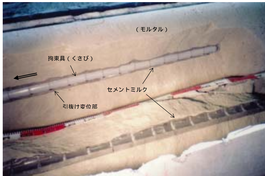
写真-2 クサビ型アンカー体定着状況 (ヒューム管 700mm 内で実施した室内実験より)
